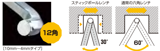
補助ハンドル
